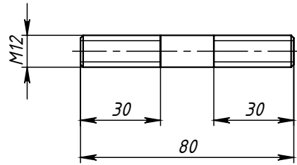
Поз.3 (Шпилька) 1:2
